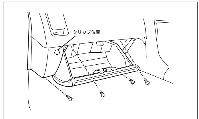
(2)グローブボックスA ssyを取外します。
